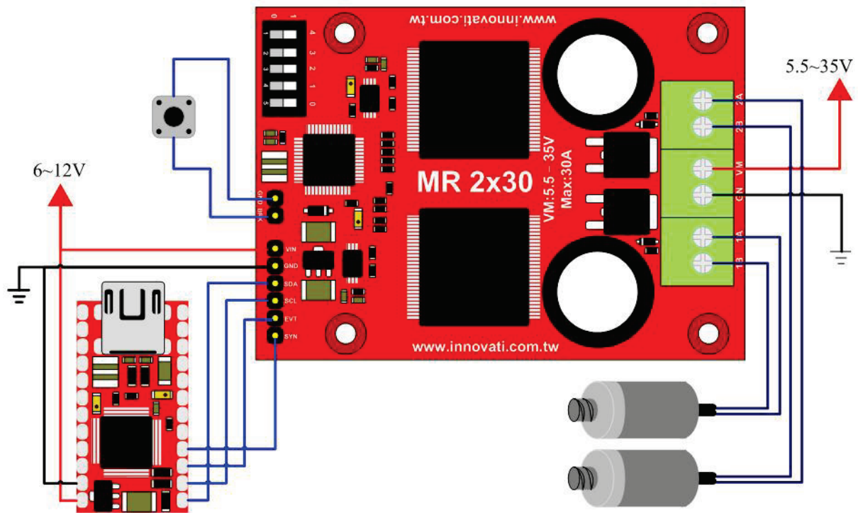
圖 1: 馬達模組連接範例
