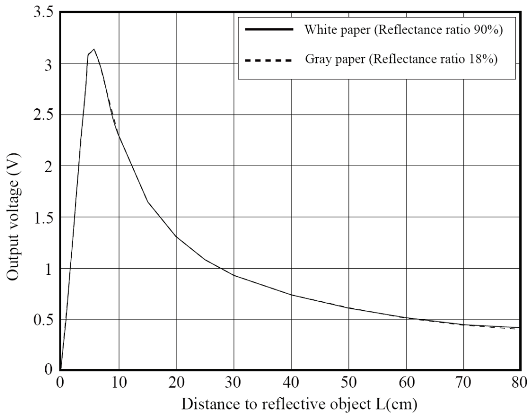
圖五:輸出距離特性圖
