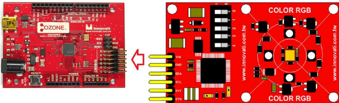
圖 1: 與 Ozone 連接
